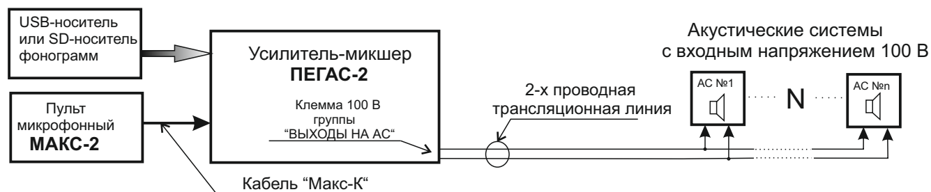
Рис.1 Схема функциональная системы “ГОЛОС”
