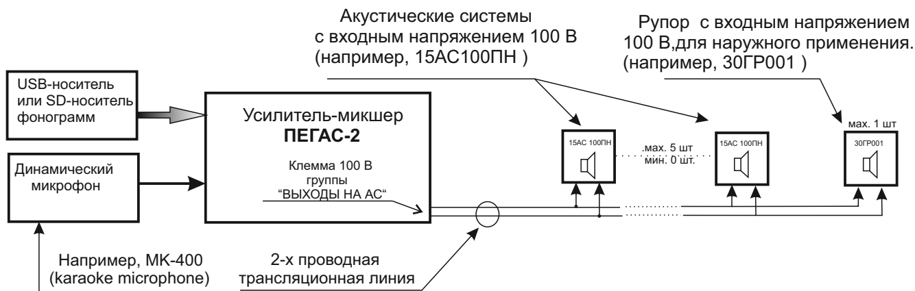
Рис.2 Схема функциональная системы “ГОЛОС” с максимальной нагрузкой по линии 100 В. (источником сигнала является только динамический микрофон и USB носитель, если нужно)
