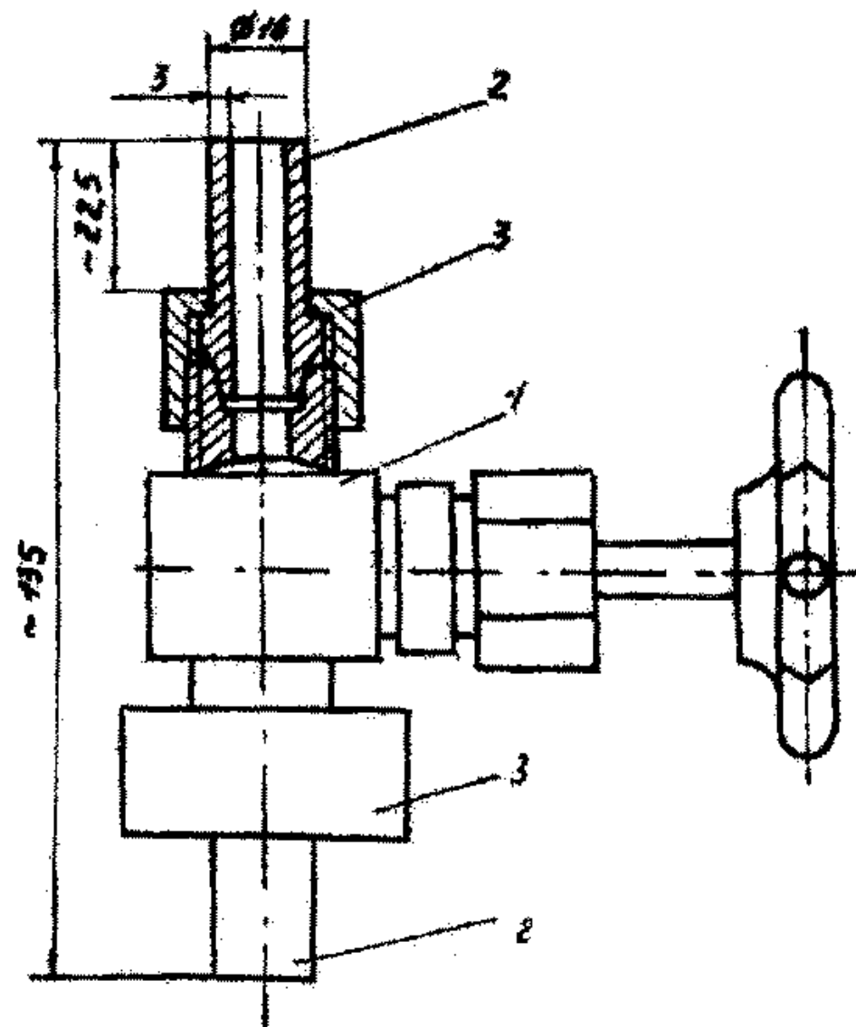
1 - клапан; 2 - ниппели; 3 - гайка
